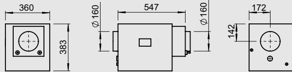
Maße in mm
